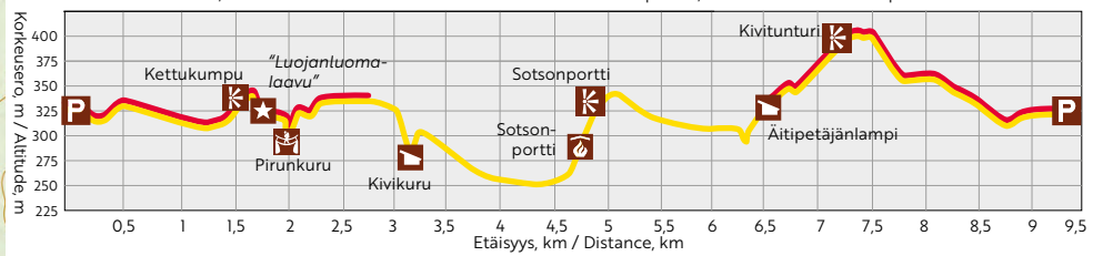
KORKEUSPROFIILI, PERUSREITTI / Route profile, basic route
